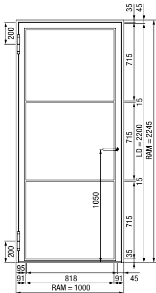
1-krilna čelična Loft vrata
