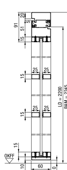
Okomiti presjek 1-krilnih čeličnih Loft vrata
