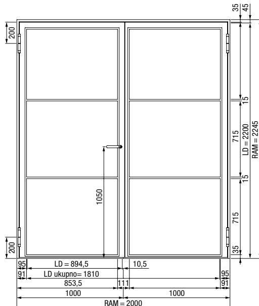
2-krilna čelična Loft vrata
